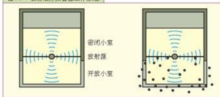
图 5.3-7 辐射烟雾报警器工作原理
