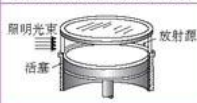
图 5.4-2 威尔逊云室结构示意图
