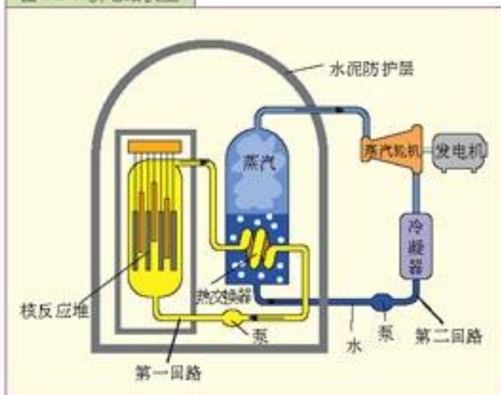
图 6.2-6 核电站模型
