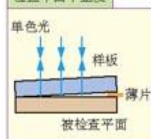
图 3.2-6 干涉法检查平面平整度
