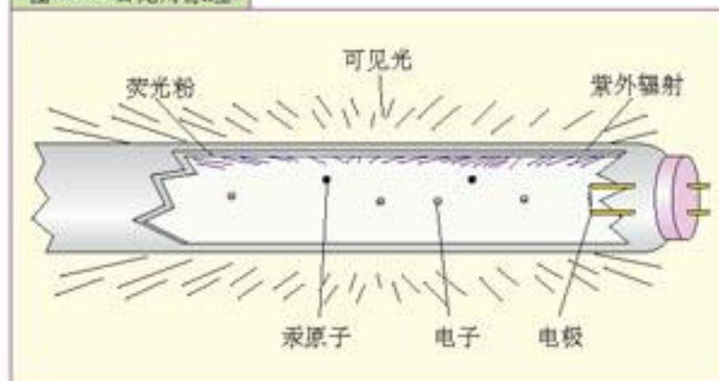
图 4.2-3 日光灯原理
