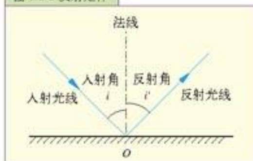
图 1.1-2 反射定律
