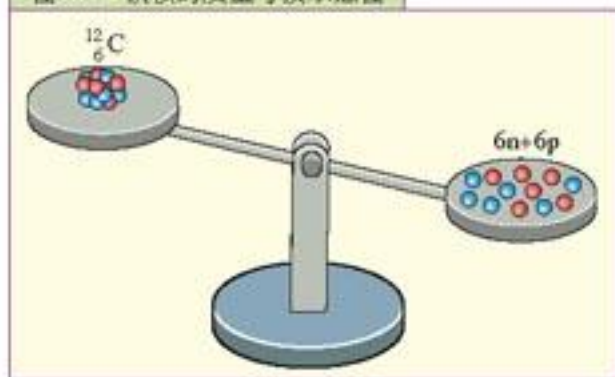
图 6.1-2 碳核的质量亏损示意图
