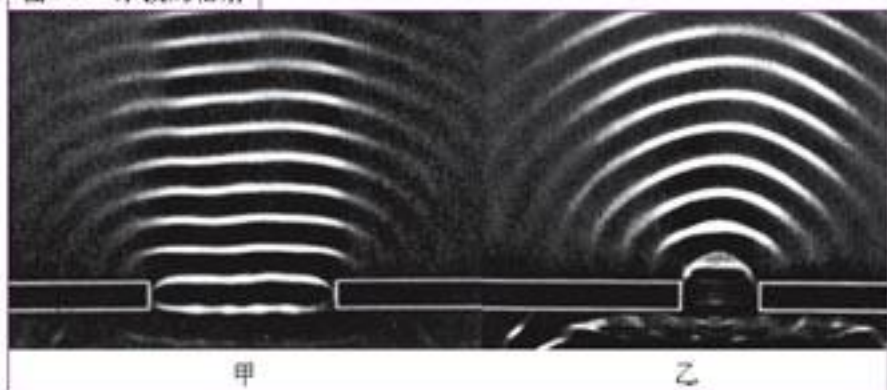
图 3.1-5 水波的衍射
