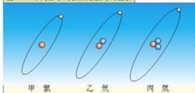
图 5.1-7 下列原子的核都是氢的同位素
