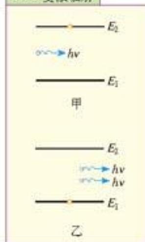
4.3-1 受激辐射
