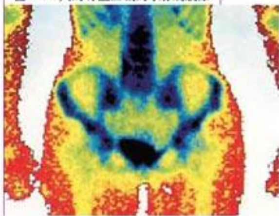
图 5.3-1 人的骨盆区域的 \gamma 射线成像
