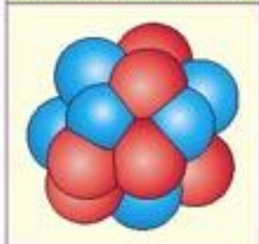
图 5.1-6 原子核的组成
