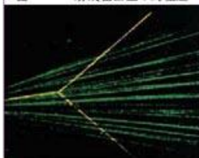
图 5.4-3 \alpha 射线在云室中的径迹
