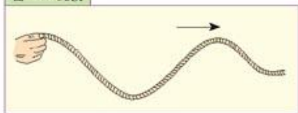
图 3.1-2 绳波
