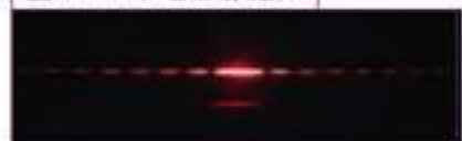
图 3.3-1 单缝衍射花样
