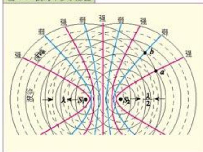
图 3.1-7 波的干涉示意图
