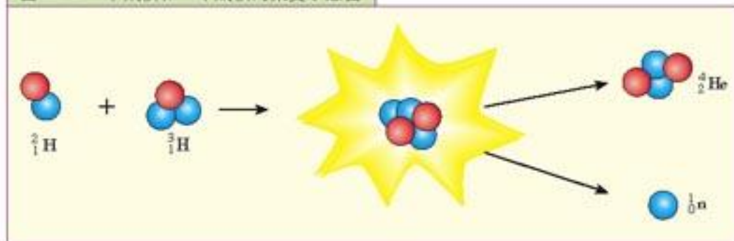
图 6.3-2 一个氘核和一个氚核的聚变示意图
