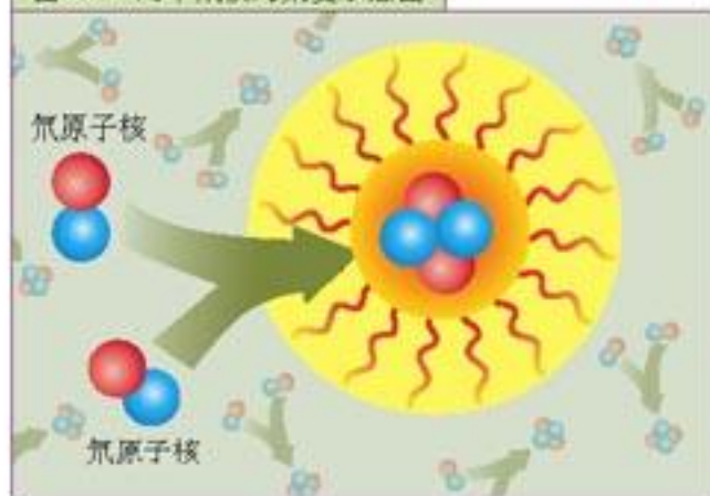
图 6.3-1 两个氘核的聚变示意图
