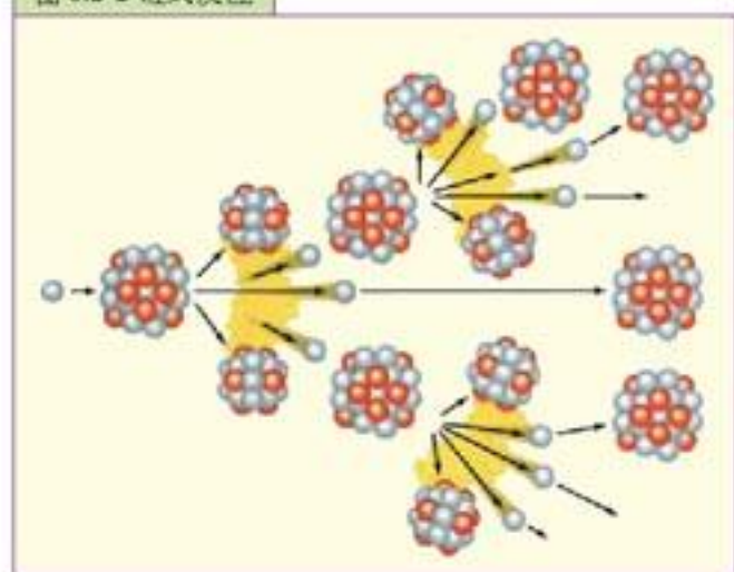
图 6.2-2 链式反应
