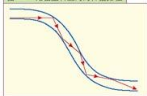
图 1.2-4 光在塑料丝内的传播路径
