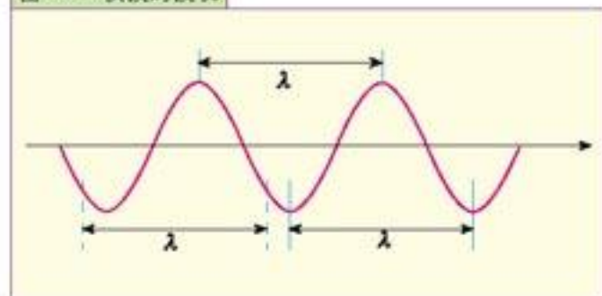
图 3.1-4 横波的波长
