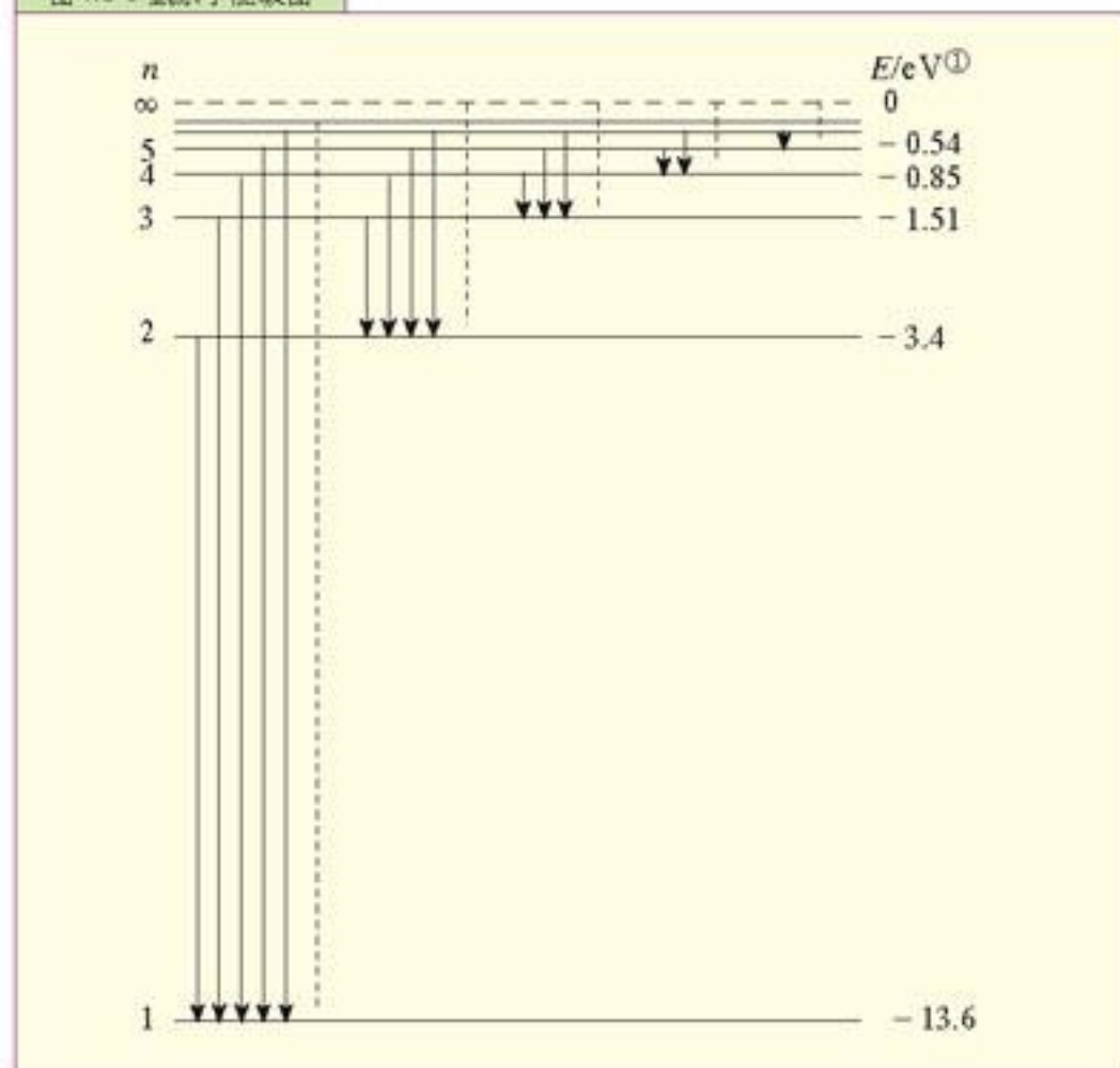
图 4.1-1 氢原子能级图
