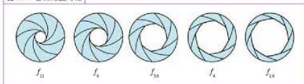
图 2.3-4 各档光圈对比
