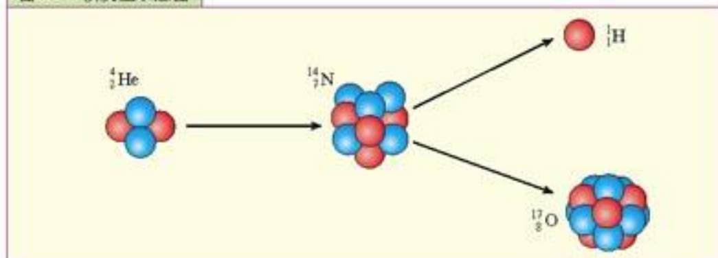
图 6.1-1 核反应示意图
