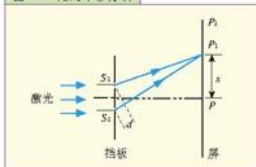
图 3.2-3 光的干涉分析
