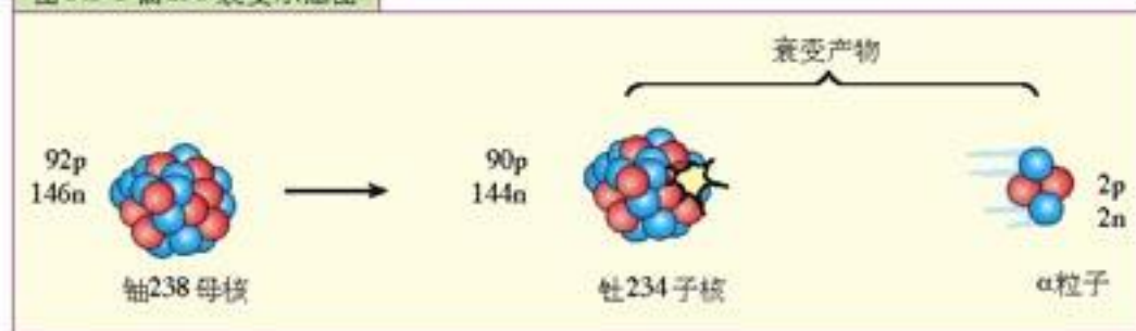
图5.2-1 铀238衰变示意图
