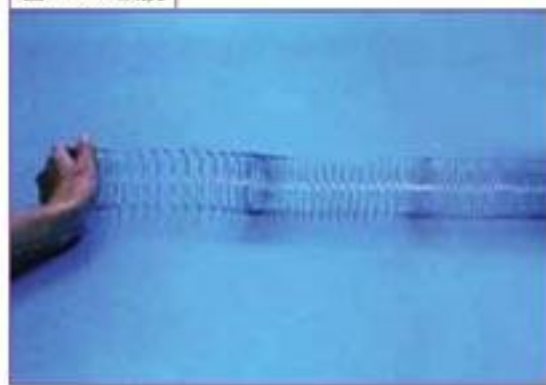
图 3.1-3 纵波
