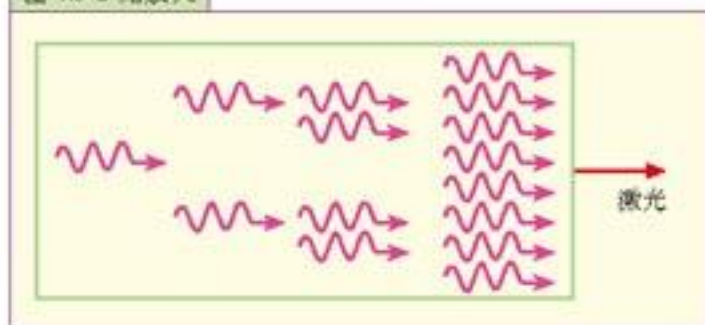
图 4.3-2 光放大
