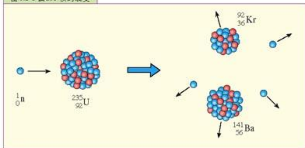
图 6.2-1 铀 235 核的裂变
