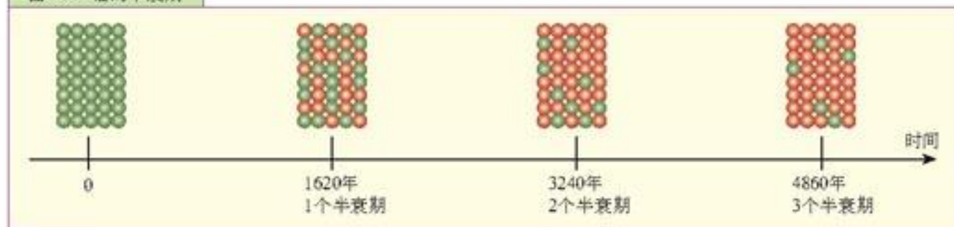
图 5.2-3 镭的半衰期
