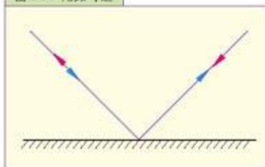
图 1.1-3 光路可逆
