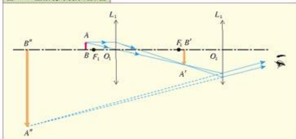
图2.2-2 显微镜的成像光路图
