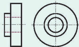
图5-25 轴套
