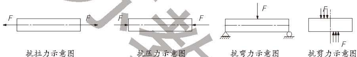
图6-11 木材受力示意图
