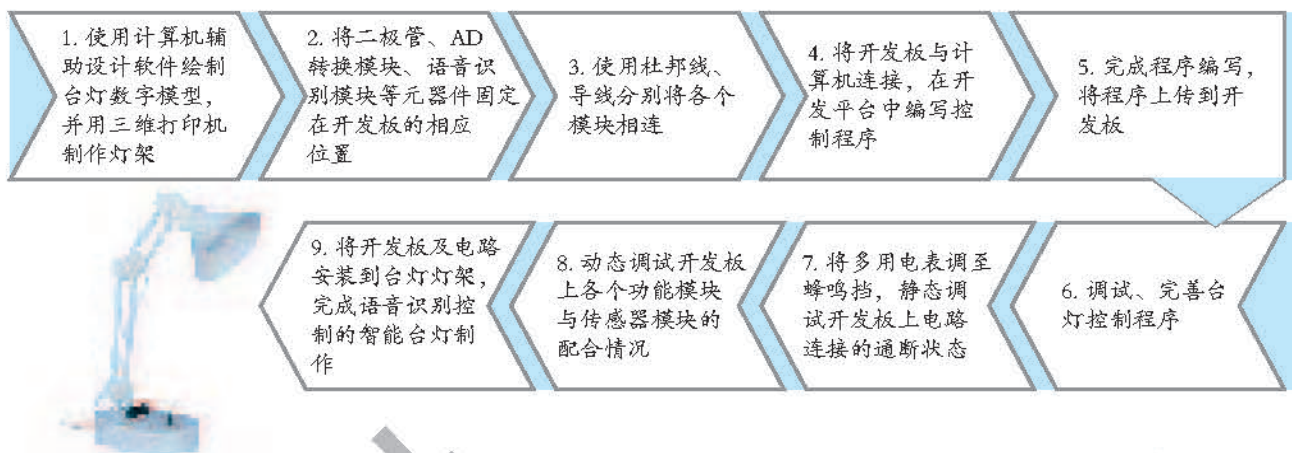
图6-56 语音识别控制的台灯
