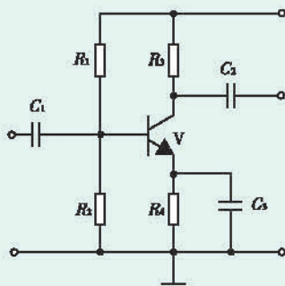
图5-32 电路图
